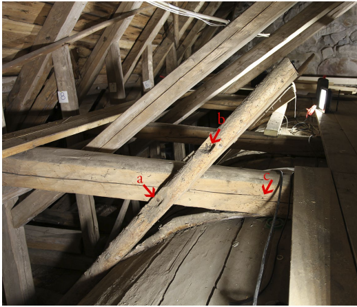
Kuva 11. Laipion rakenteen muutos näkyy selkeästi lähes kaikissa ruoteissa. Kuva pohjoispuolen neljännessä ruoteesta idästä lukien. a) nykyinen naulaus, b) aiempi naulan kolo ruoteessa, c) naulanreikä laipion niskassa. Kuva: Laura Laine.
