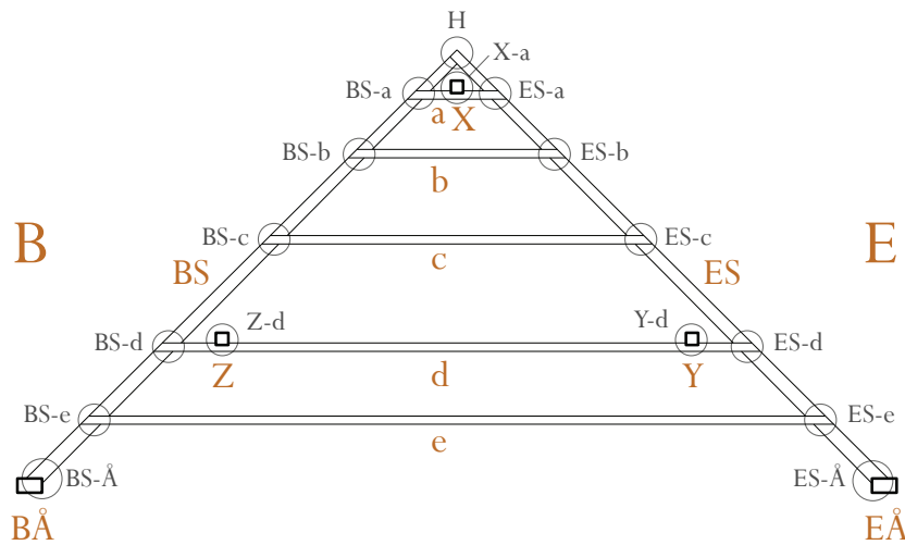
Louhisaaren kaakkoisen sivurakennuksen lautakatteen limitys ja nykyinen harjan rakenne.
