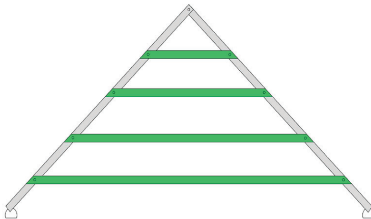
Puristettu kattotuoli
