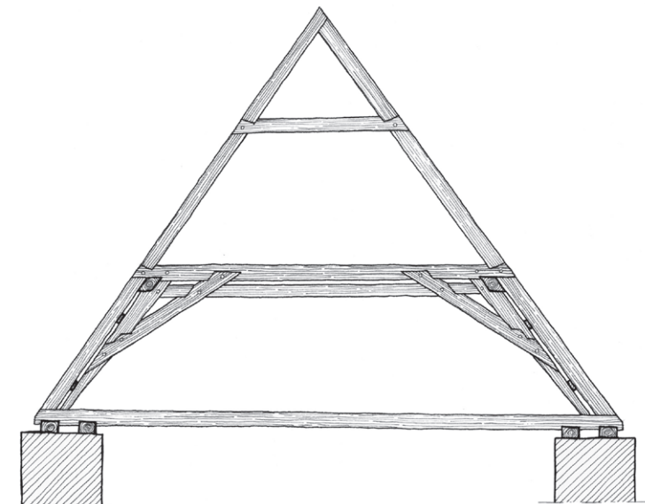
Pukkirakenteen periaate.
