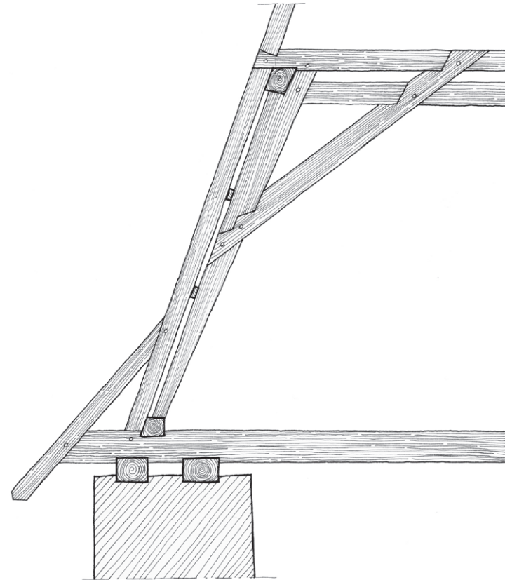
Hollantilainen räystäsrakenne.
