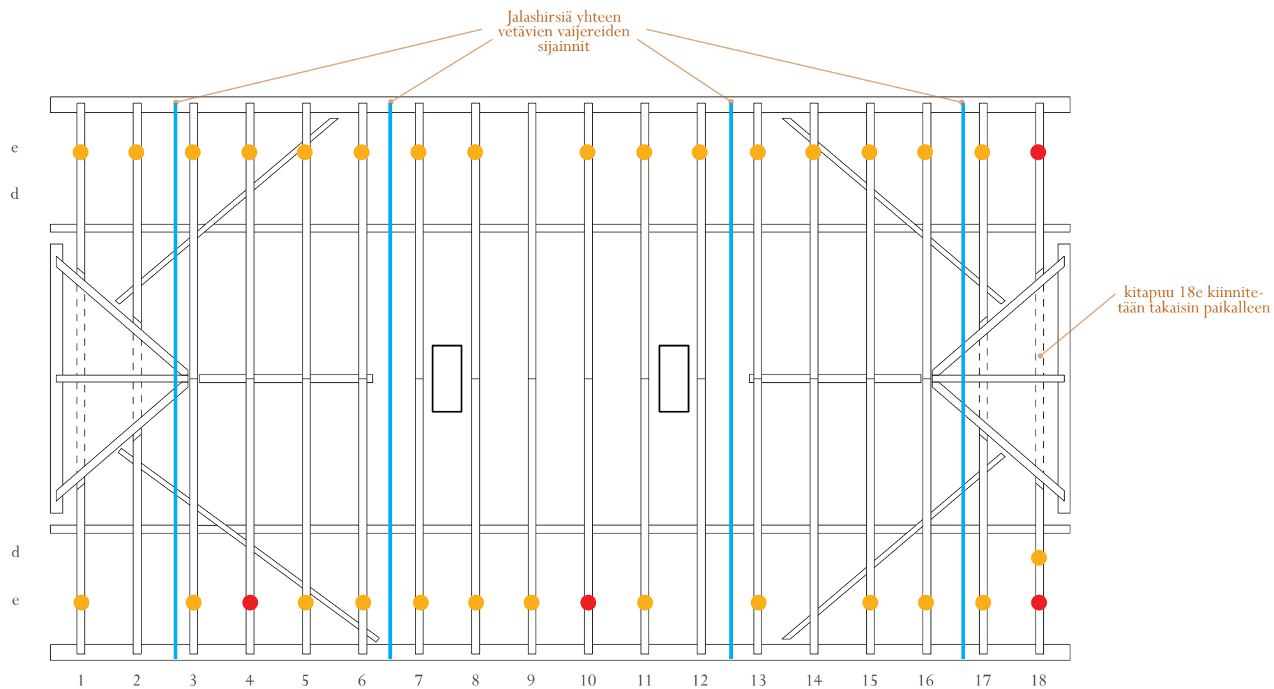
Kantavan kattorakenteen restauroinnin palauttava vaihtoehto (B) 1:100.
