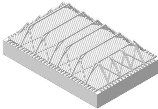
5. Pukkirakenteen jäykistys saksipuvin.
