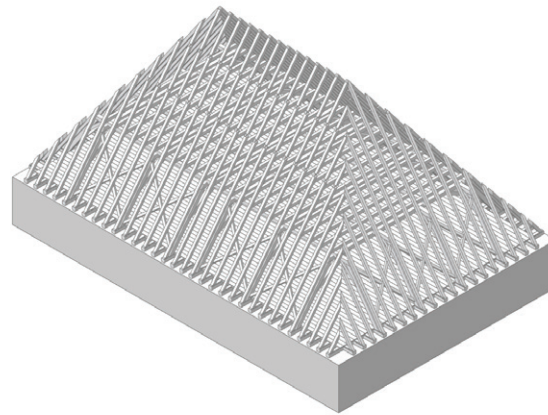
8. Selkämpuiden pystyttäminen ja ylimpien kitapuiden (a ja b) kiinnittäminen lapaliitoksiin.
