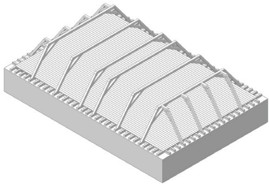
4. Pukkirakenne.
