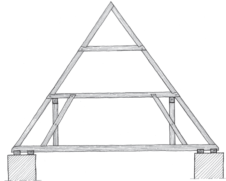
Kaksitukisen piirukaton rakenneperiaate.
