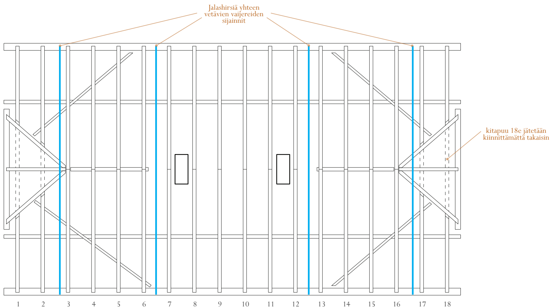
Kantavan kattorakenteen restauroinnin nykytilanteen säilyttävä vaihtoehto (A) 1:100.
