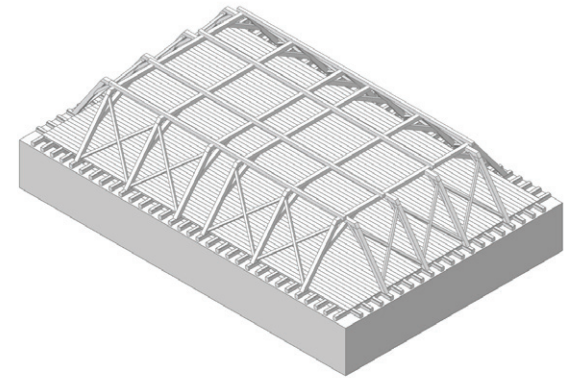
6. Vuoliaisten asettaminen pukkien päälle.
