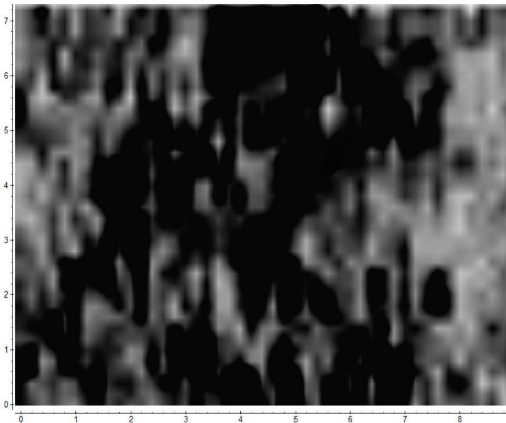
Kuva 2. Ote kohteen K1 amplituditasokartasta Reflexw-ohjelmistolla visualisoituna. Kuva: T. Väisänen.
