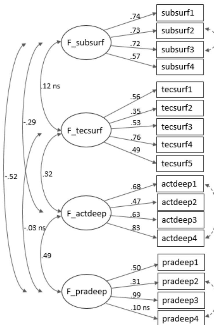
Kuva 1. CFA-mallin estimointitulokset.
