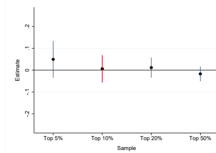
(e) GPA
