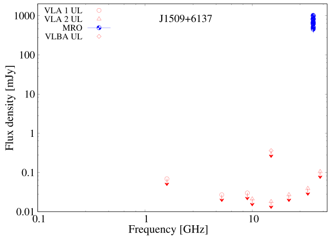
(d) Non-simultaneous radio spectrum of J1509+6137.
