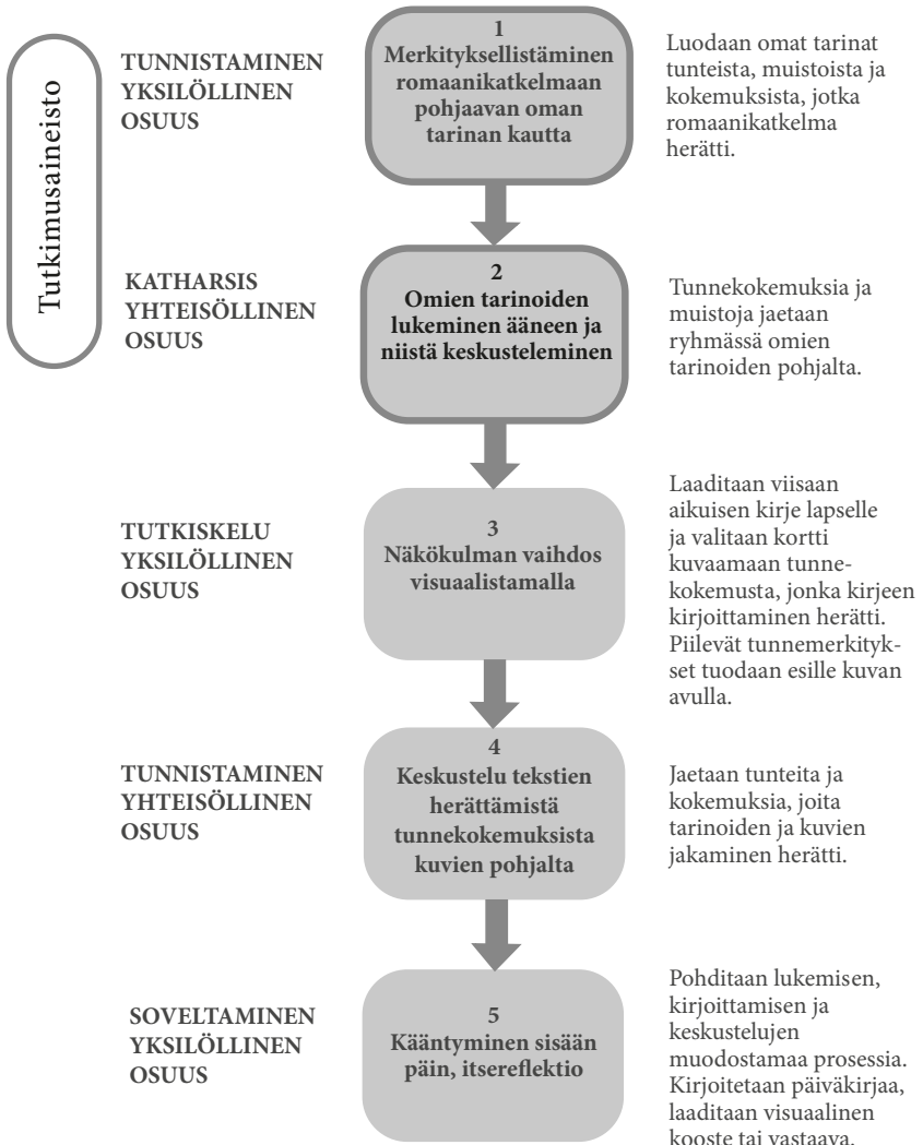
Kuvio 2. Eläytyvän lukemisen prosessimalli koulutukseen (mukaillen Kauppinen & Aerila 2024).
