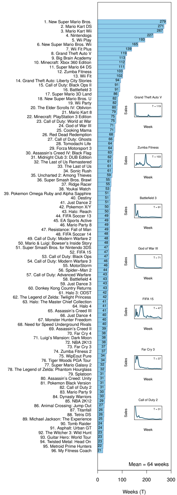
Fig. 3 The Dataset
