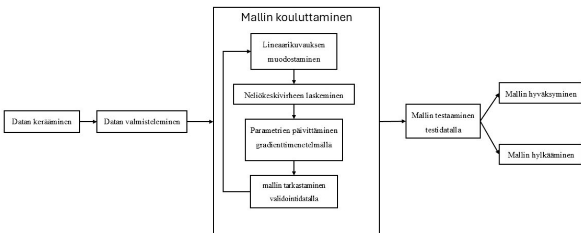
Kuva 3: esimerkki vuokaaviosta.
