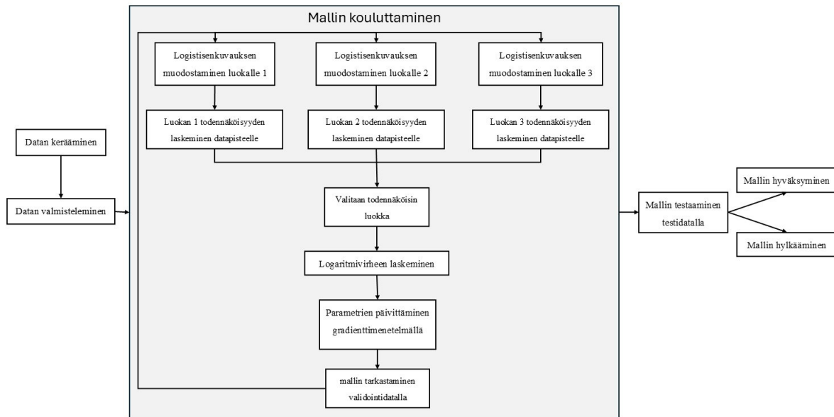
Kuva 9: Esimerkki logistisen regressioon vuokaaviosta
