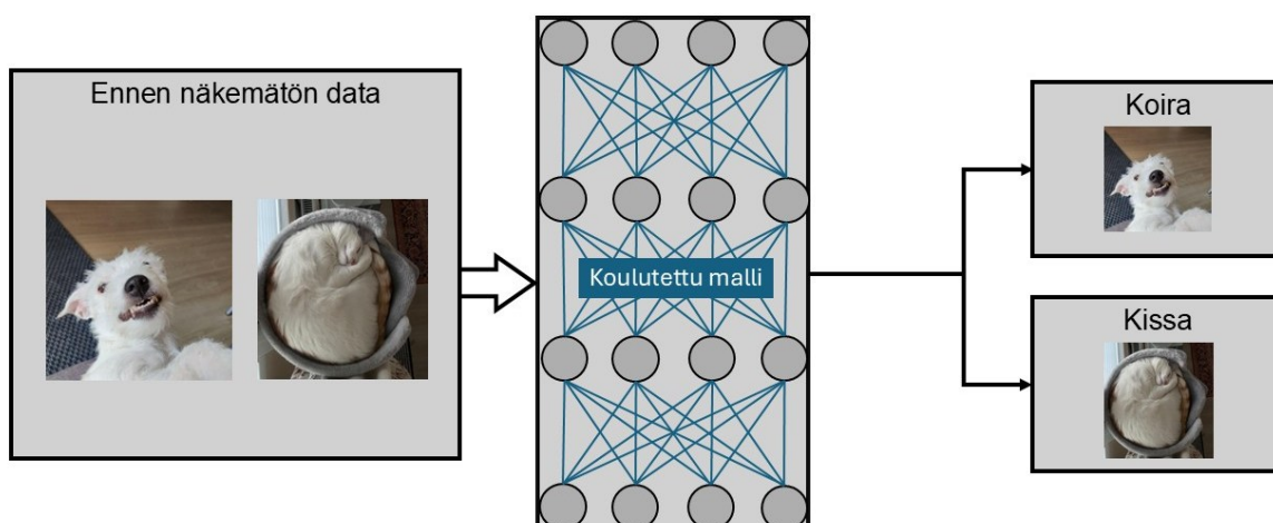
Kuva 5: Koulutettu luokittelumalli.
