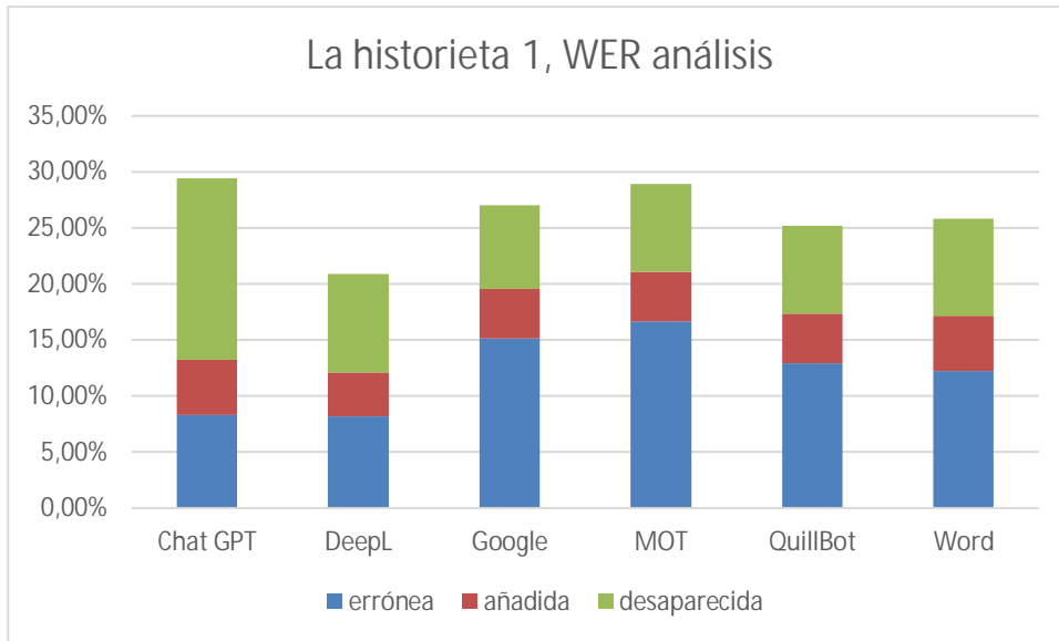
Ilustración 3, La historieta 1, WER análisis. Las cuotas de las palabras erróneas, añadidas y desaparecidas
