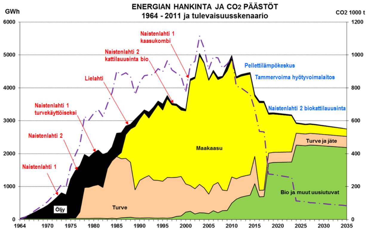
Kuva 3. Tampereen Sähkölaitoksen energian hankinta ja CO 2 päästöt (1964–2011) ja tulevaisuusskenaario. Kehitysohjtaja Mika Pekkinen Tampereen Sähkölaitos Oy, 2013.
